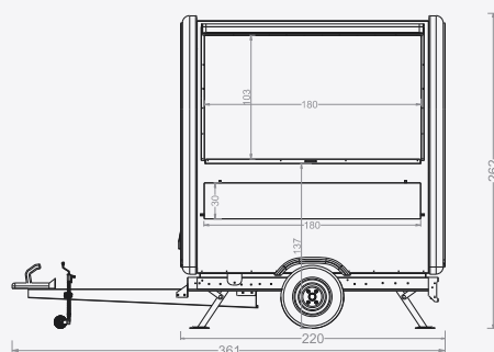
PROFIL, CÔTÉ SERVICE
