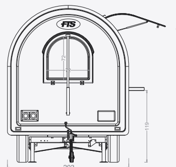
FACE AVANT
